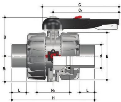
Шаровой кран VKD ПВДФ с втулочными окончаниями, DN65-100 d110 (DN100)
