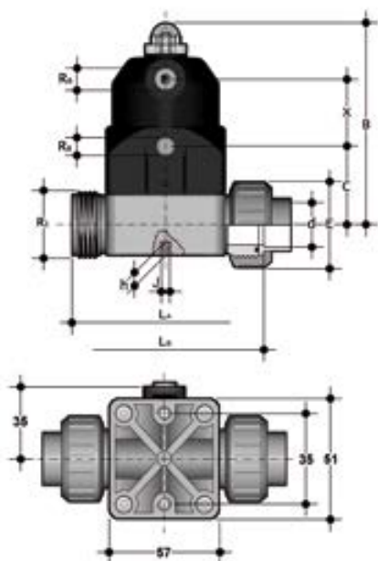
Компактный мембранный клапан CM с пневмоприводом НЗ с муфтовыми окончаниями (уплотнение EPDM/мембрана EPDM) PP-H d16 (DN12)
