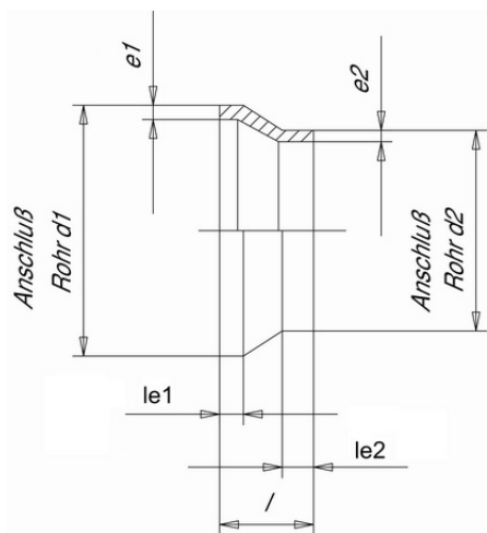
Муфта редукционная ПВДФ (Simona) 125x110 SDR21 PN16
