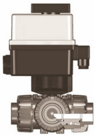
3-х ходовой шаровой кран TKD ХПВХ с эл.приводом 90-240V, муфтовые окончания, L-шар d50 (DN40)
