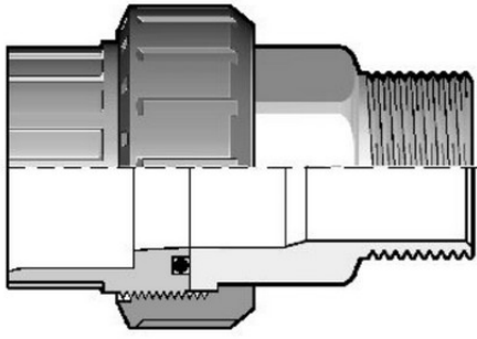
Муфта разборная переходная ХПВХ/ нержавеющая сталь НР 16x3/8" PN16
