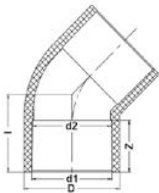
Отвод 45° ХПВХ IPS (Model B) d140 PN16
