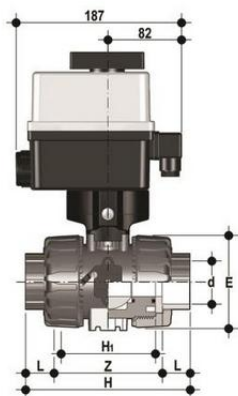
Шаровой кран VKD ХПВХ с эл.приводом 24V AC/DC, муфтовые окончания d63 (DN50)
