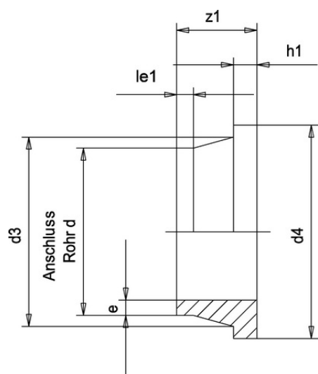
Бурт ПВДФ (Simona) d75 SDR21 PN16
