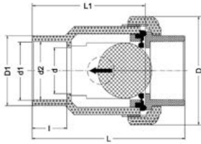
Обратный клапан шаровой с одним разборным соединением, муфтовые окончания PP-H IPS (EPDM) d40 (DN32)
