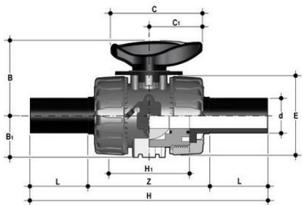
Шаровой кран ПВХ для регулирования потока VKR с патрубками из ПЭ , EPDM, FIP d40 (DN32)
