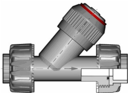
Угловой обратный клапан VRUIV ПВХ с разборными муфтовыми окончаниями, FKM, FIP d63 (DN50)
