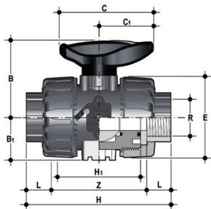
Шаровой кран промышленного применения VKD с резьбовыми окончаниями (уплотнение EPDM) PP-H R1/2" (DN15)
