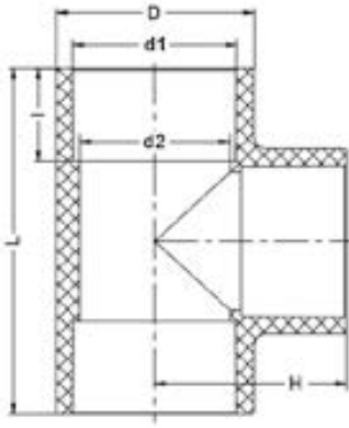
Тройник ПВДФ для раструбной сварки 90° d75 PN 16
