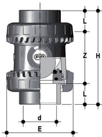
Шаровой обратный клапан SXE ХПВХ с муфтовыми окончаниями d32 (DN25)
