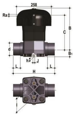
Мембранный клапан DK ПВХ с пневмоприводом, PN10, фланцевые окончания, EPDM, FIP d90 (DN80)
