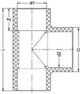
Тройник 90° ХПВХ IPS (Model B) d355 PN10
