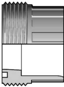
Муфтовая вставка ХПВХ d25 PN16
