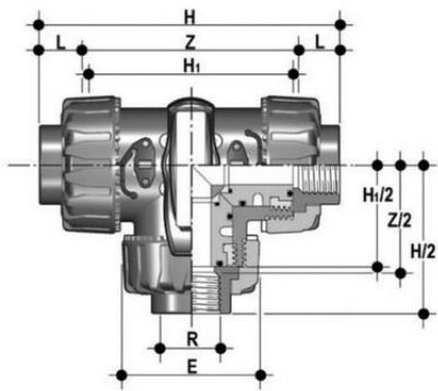
3-х ходовой шаровой кран ТКД с резьбовыми окончаниями Т-шар (уплотнение FKM) PP-H R1¼" (DN32)
