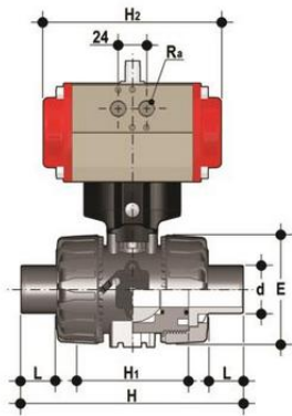
Шаровой кран VKD с пневмоприводом ДвД с удлинёнными патрубками ПП (уплотнение FKM) PP-H d20 (DN15)
