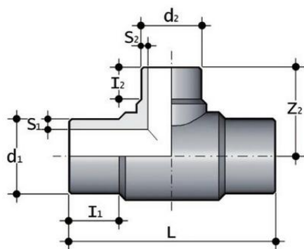
Тройник редукционный для стыковой сварки PP-H FIP (PN10) 160x125 SDR11 PN10
