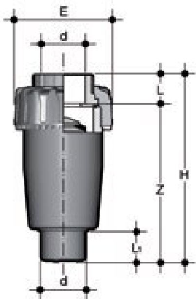
Воздухоотводный клапан VA ПВХ с муфтовыми окончаниями, EPDM, FIP d20 (DN15)
