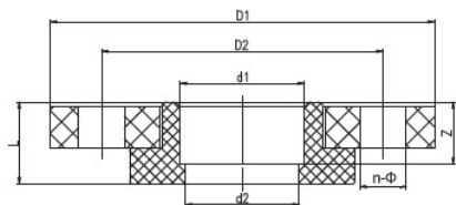
Бурт+фланец (комплект) для раструбной сварки РР-Н IPS d110 PN10
