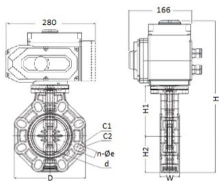
Дисковый затвор IFK ПВХ с электрическим приводом 24V DC, FKM, IPS d160 (DN150)
