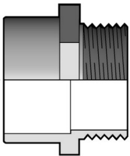
Адаптер с наружной резьбой PP-H FIP 25x3/4 SDR11 PN6
