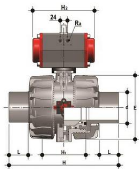
Шаровой кран VKD ПВХ с пневмоприводом ДвД с втулочными окончаниями, EPDM, FIP d90 (DN80)
