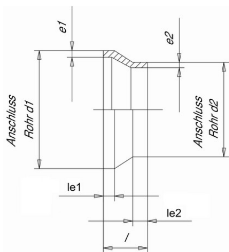
Муфта редукционная PP-H Simona 315x200 SDR11 PN6
