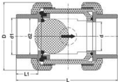
Шаровой обратный клапан ISXE ПВХ; с муфтовыми окончаниям, EPDM, IPS d25 (DN20)
