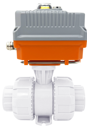
Шаровой кран IVKD ПВДФ с эл.приводом 220V AC, муфтовые окончания, FKM, IPS d90 (DN80)
