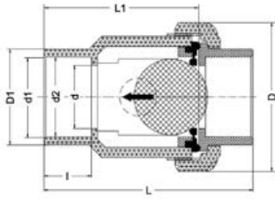
Обратный клапан шаровой с одним разборным соединением, муфтовые окончания PP-H IPS (EPDM) d75
