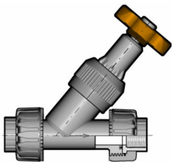
Угловой вентиль VVUFV PBX с резьбовыми окончаниями, EPDM, FIP R1¼" (DN32)
