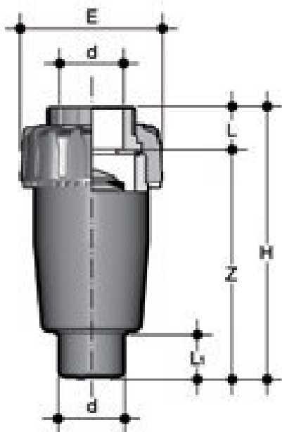
Воздухоотводный клапан VA PBX с муфтовыми окончаниями, EPDM, FIP d40 (DN32)
