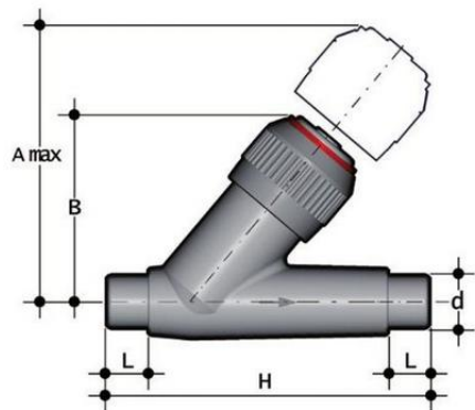
Угловой обратный клапан VRDV ПВХ с втулочными окончаниями, EPDM, FIP d63 (DN50)
