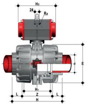
Шаровой кран VKD ПВДФ с пневмоприводом НО с муфтовыми окончаниями d75 (DN65)
