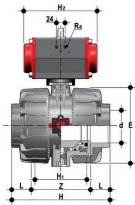
Шаровой кран VKD ПВХ с пневмоприводом ДвД с муфтовыми окончаниями, FKM, FIP d75 (DN65)
