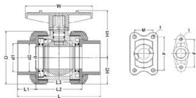
Шаровой кран IVKD ПВДФ с муфтовыми окончаниями d50 (DN40)
