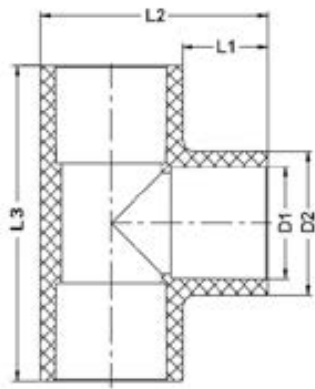
Тройник 90° ХПВХ IPS (Model A) d140 PN16
