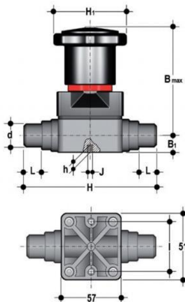
Компактный мембранный клапан ПВХ с пневмоприводом, CM, EPDM, FIP d20 (DN15)
