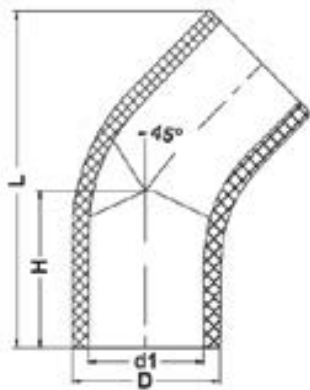
Отвод для стыковой сварки 45° PP-H IPS (Model A) d50 PN10
