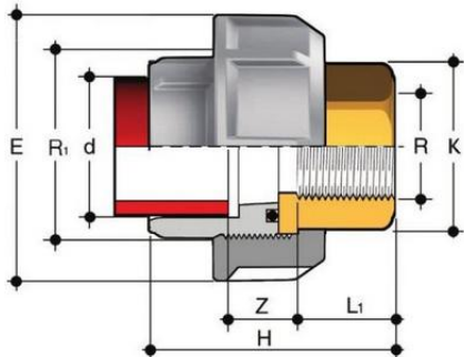
Муфта разборная переходная РР-Н / латунь, ВР (EPDM) FIP 50x1 1/2 PN10
