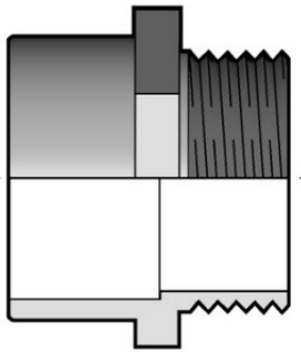
Адаптер с наружной резьбой PP-H FIP 40x1 SDR11 PN6
