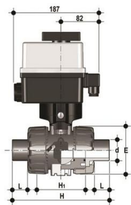
Шаровой кран VKD ХПВХ с эл.приводом 90-240V, втулочные окончания, DN65-100 d90 (DN80)
