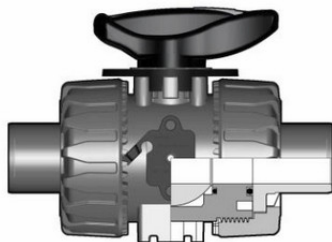
Шаровой кран для регулирования потока VKRDM с муфтовыми окончаниями (уплотнение FKM) PP-H d32 (DN25)
