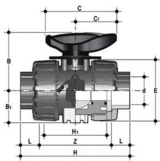
Шаровой кран ПВХ для регулирования потока VKR с муфтовыми окончаниями, EPDM, FIP d16 (DN10)
