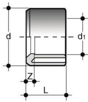
Кольцо переходное ПВХ FIP 40x20
