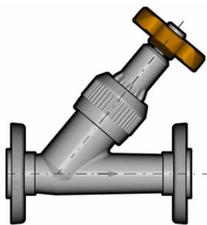
Угловой вентиль VVOV PBX с фланцевыми окончаниями, EPDM, FIP d25 (DN20)
