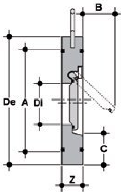
Межфланцевый обратный CROV ПВХ, EPDM, FIP d63 (DN50)
