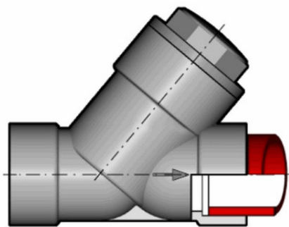
Угловой обратный клапан VR с муфтовыми окончаниями, (уплотнение FKM) PP-H d75 (DN65)
