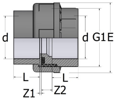
Муфта разборная ПВХ клеевая Comer d16
