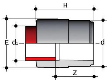
Муфта редукционная для раструбной сварки PP-H FIP 40x25 PN10
