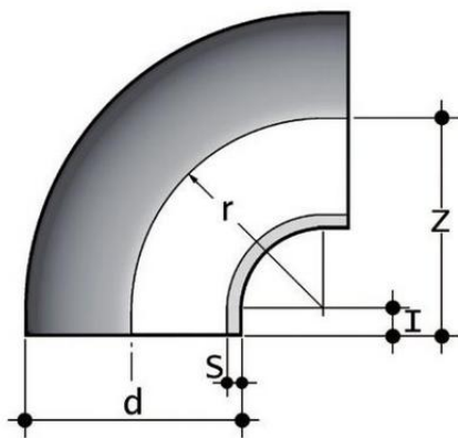
Отвод 90° для стыковой сварки PP-H FIP (PN6) d225 SDR17.6 PN6
